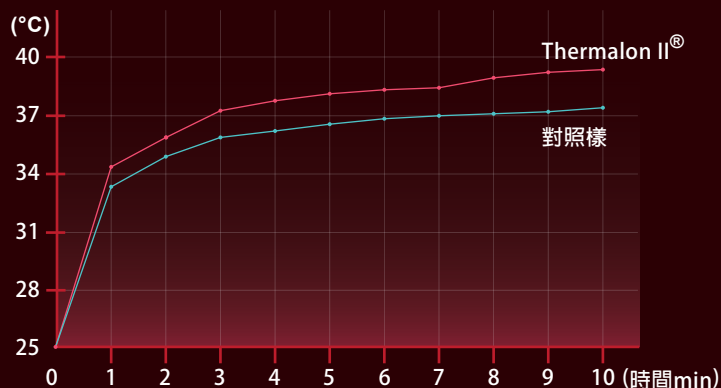
Thermalon II® 溫升曲線圖 500W鹵素燈 照射10分鐘
